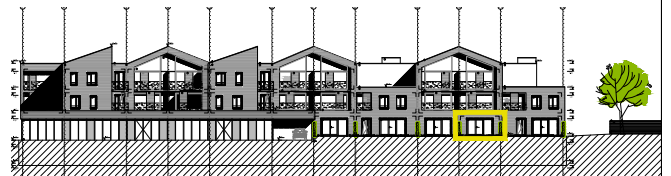
BLOK A/B Voorgevel zuid 1/1000
