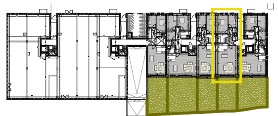
BLOK A/B Grondplan niveau +0 1/1000
